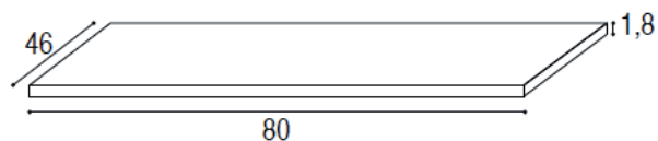
KL45/80H25C+TOP)
