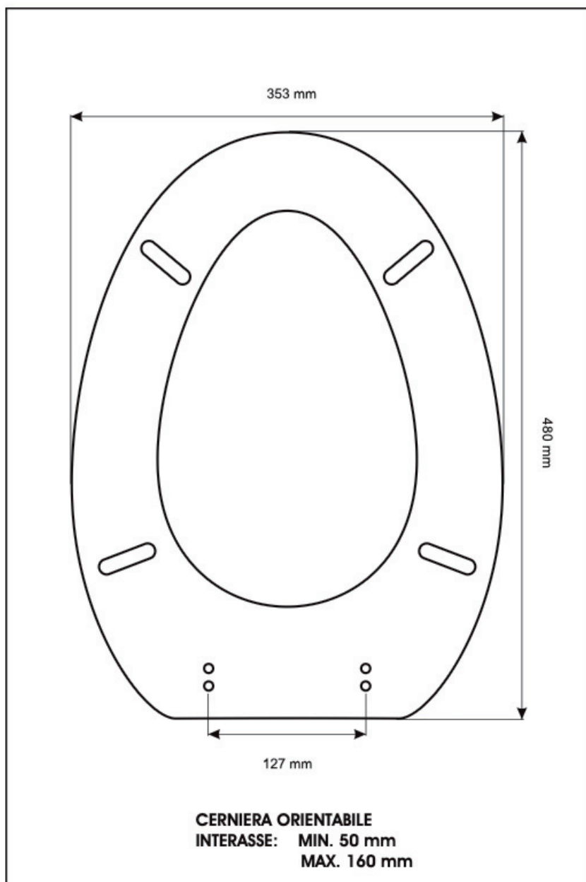
CERNIERA
